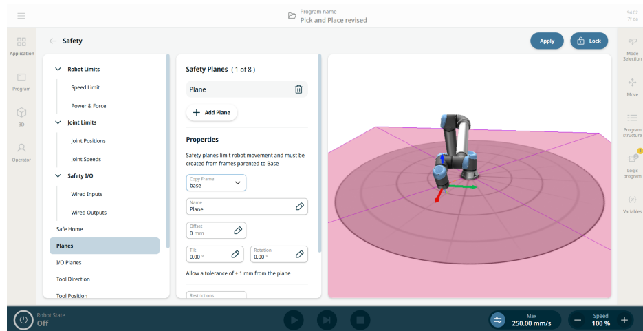
Figuur 1.5: PolyScope X-scherm met veiligheidsvlakken.
